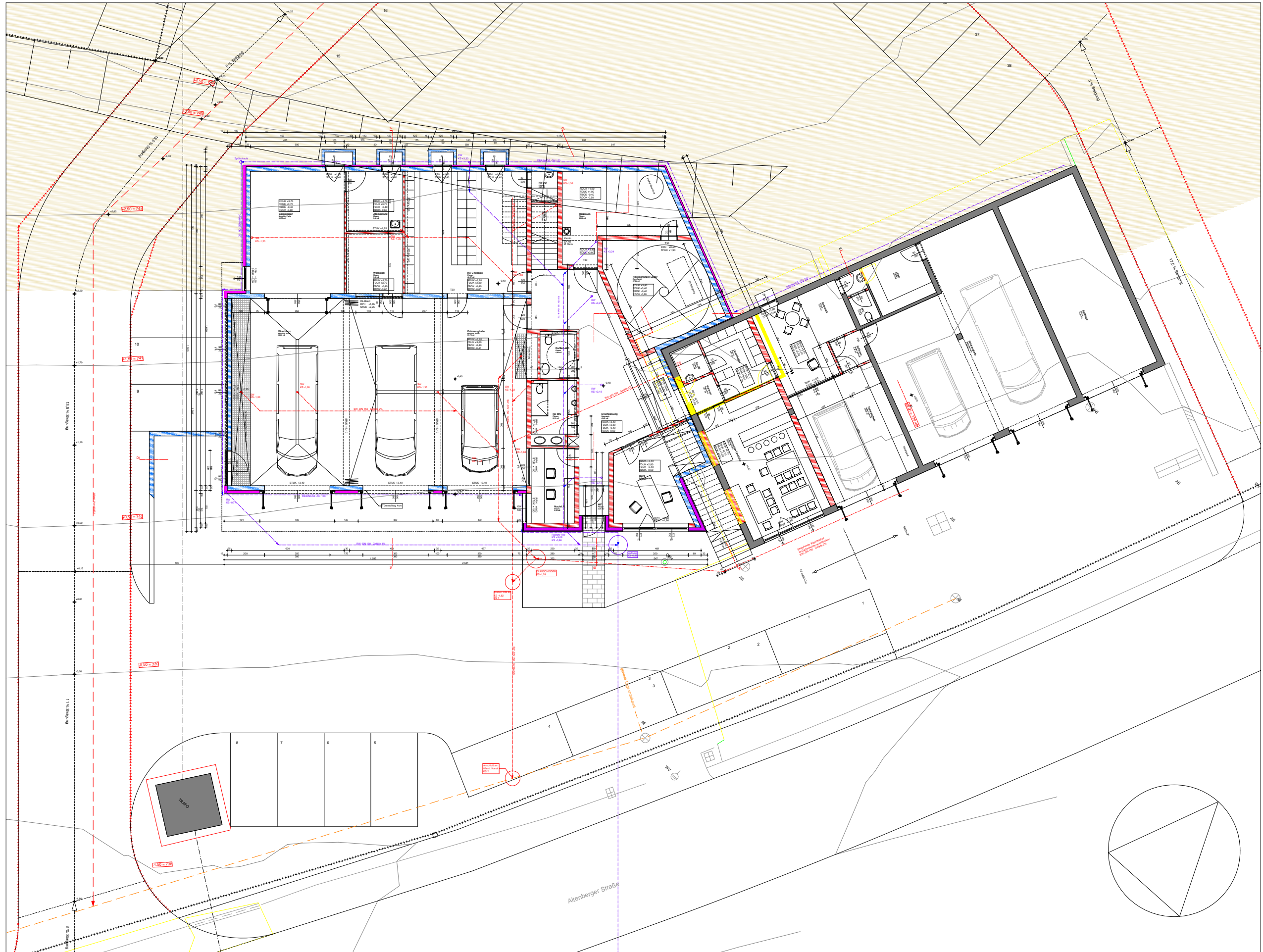
GRUNDRISS ERDGESCHOSS 1:100
