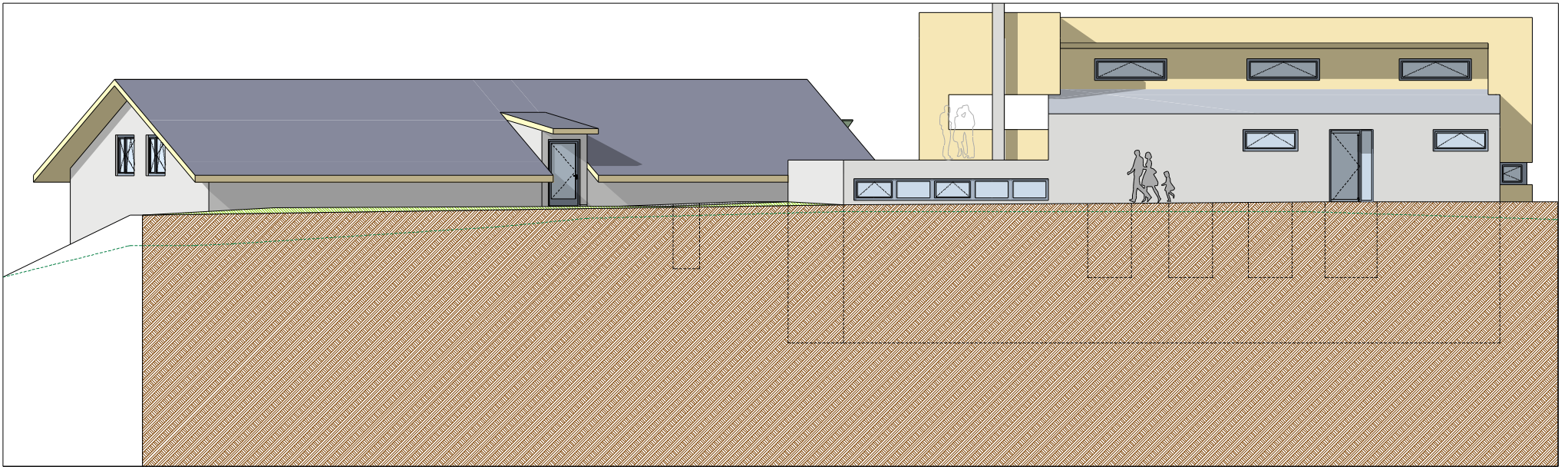
NORDWESTANSICHT 1:100
