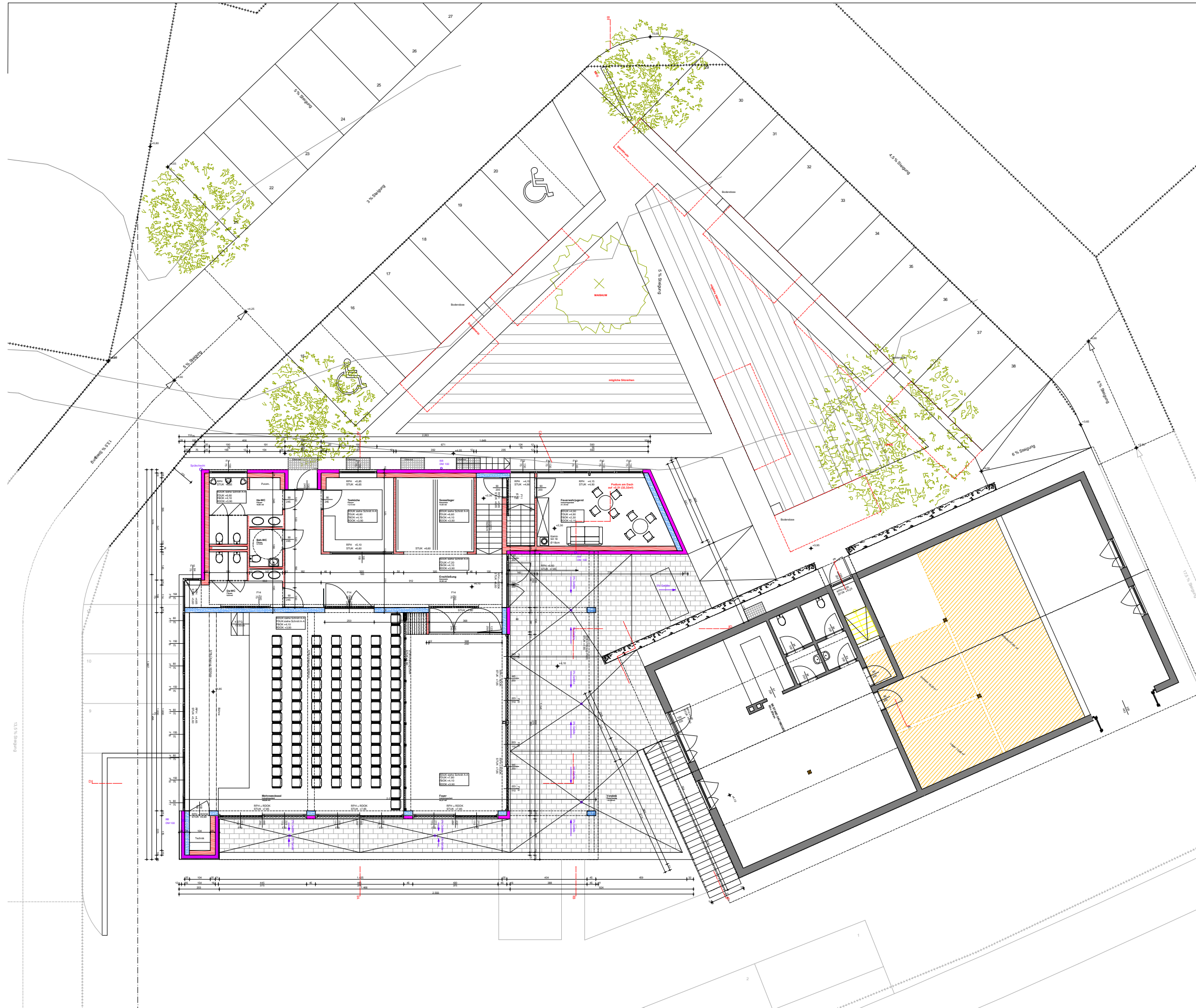
GRUNDRISS OBERGESCHOSS 1:100
