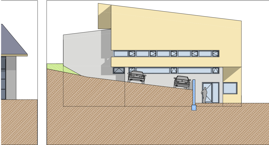
SÜDWESTANSICHT 1:100
