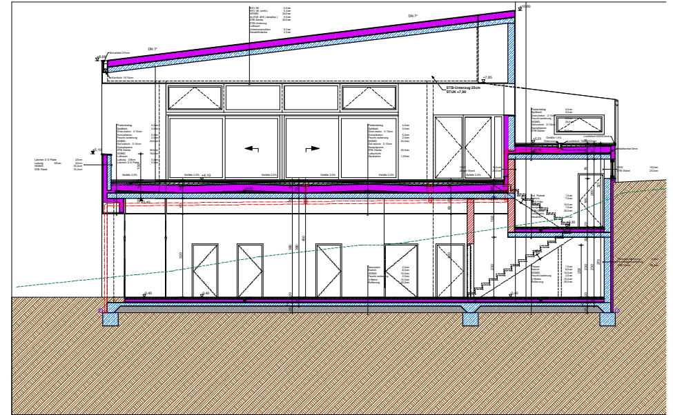
SCHNITT B-B 1:100
