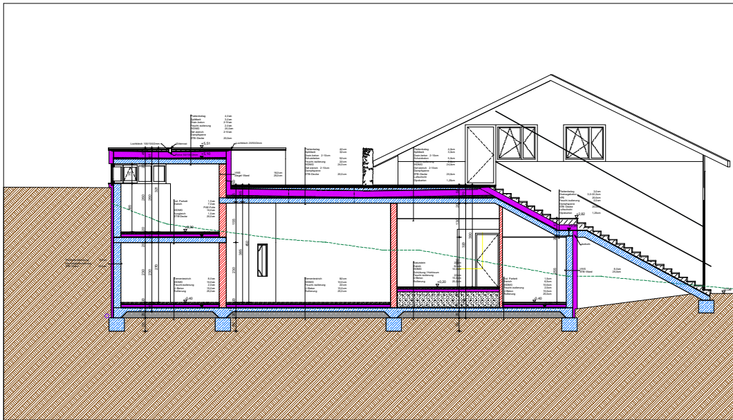
SCHNITT C-C 1:100
