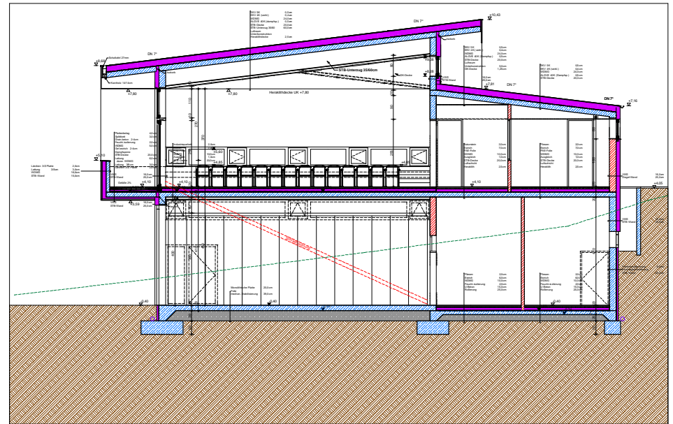
SCHNITT A-A 1:100
